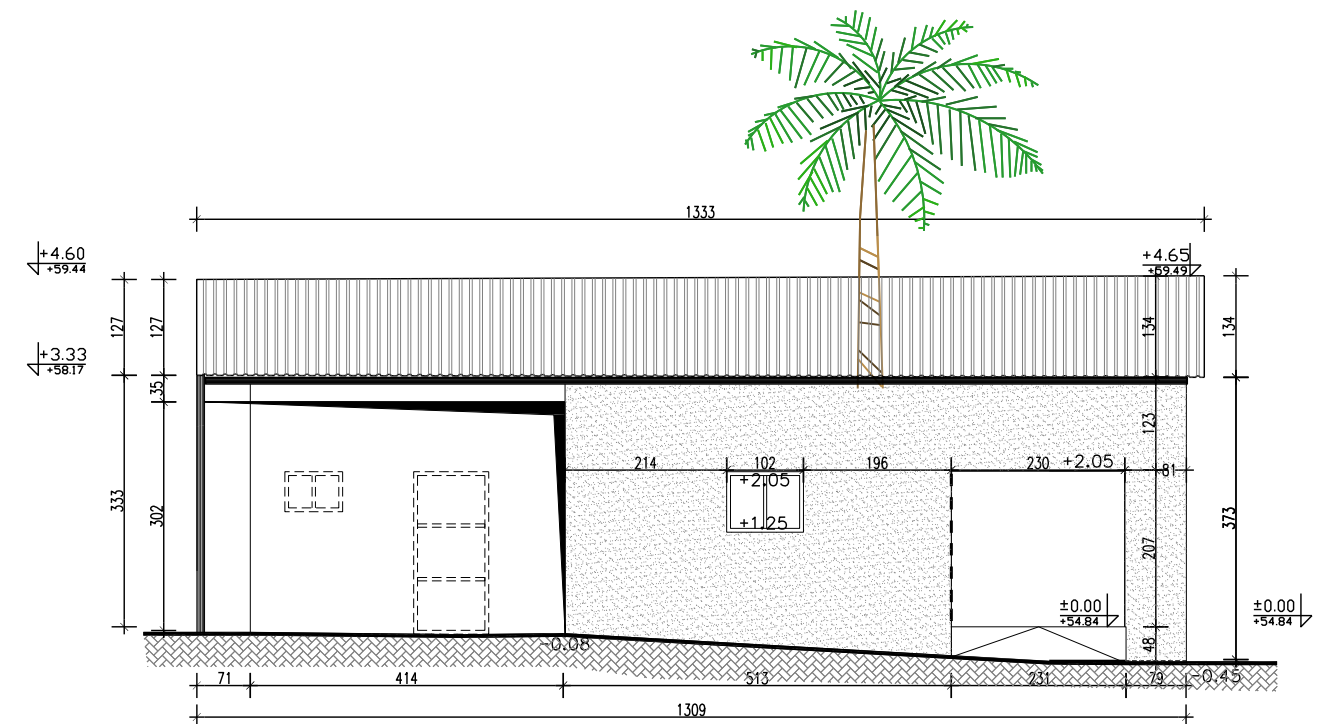
חזית דרומית - מצב מקורי משוחזר - בית משפחת יפה קנה מידה 1:100
