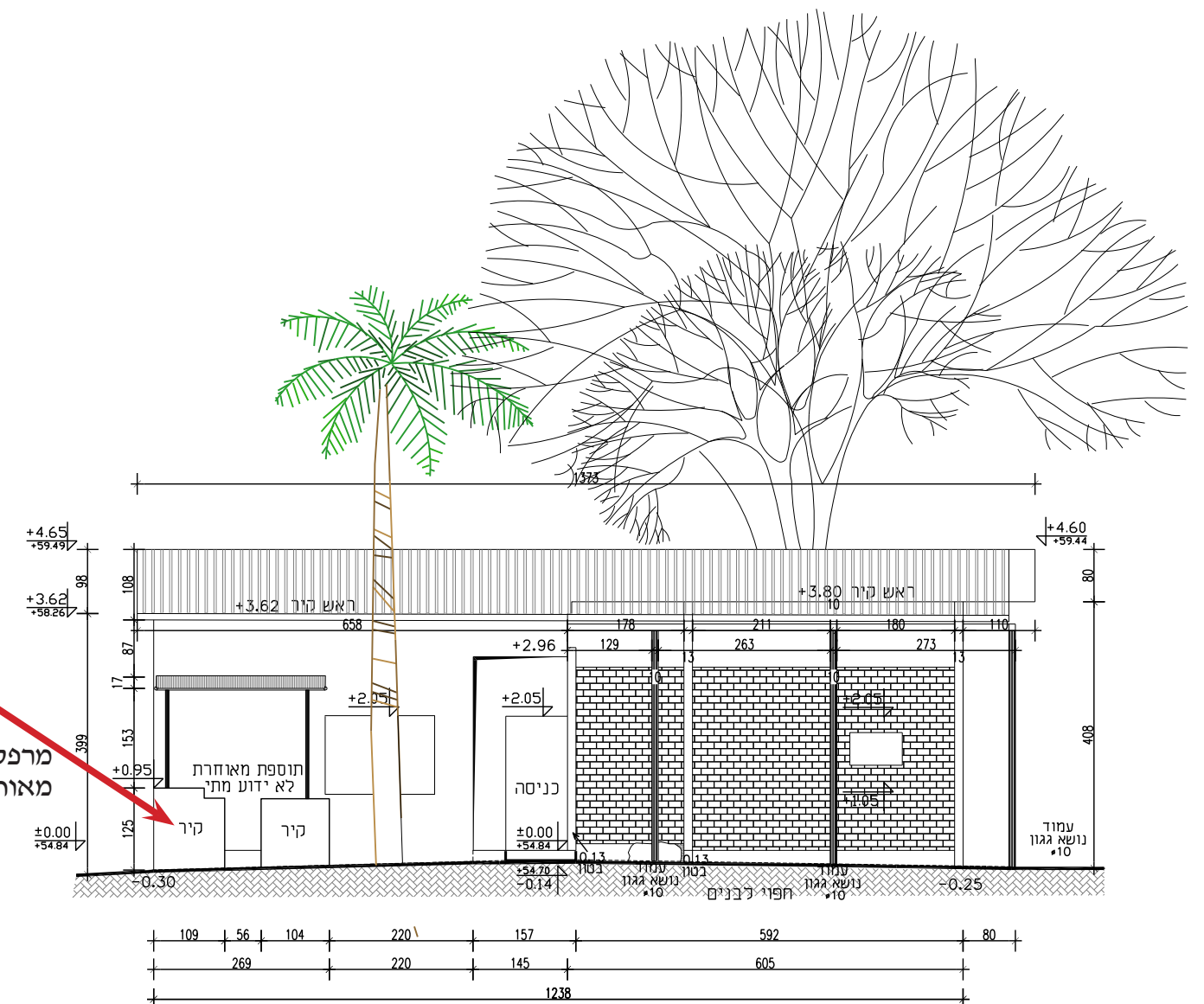
חזית צפונית - מצב מקורי משוחזר - בית משפחת יפה קנה מידה 1:100
