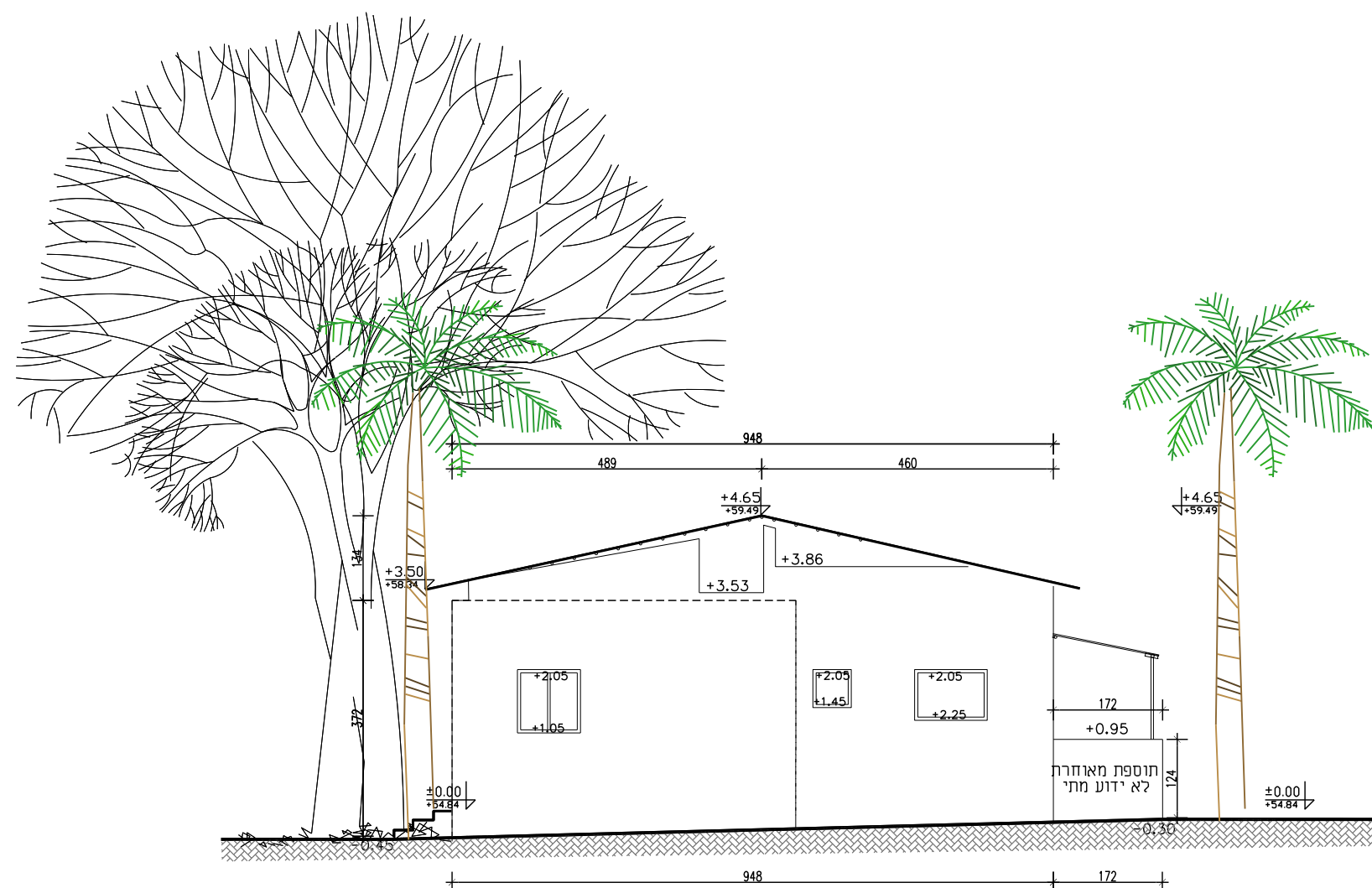
חזית דרום מזרחית - מצב מקורי משוחזר - בית משפחת יפה קנה מידה 1:100
