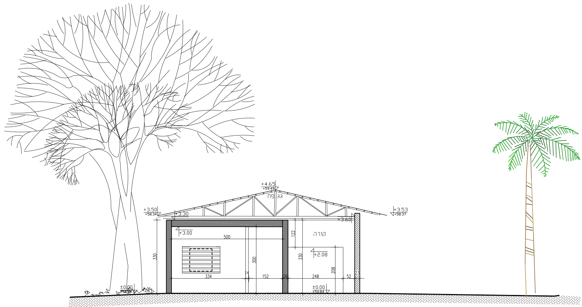
חתך ב-ב קנה מידה: 1-100
