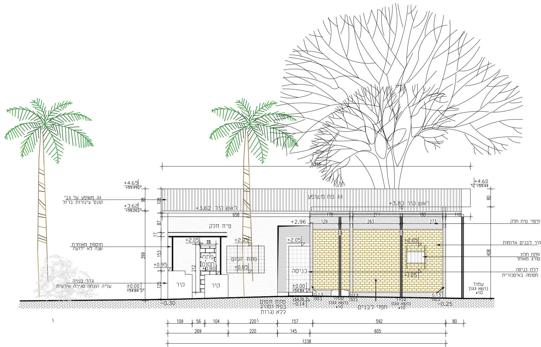
חזית צפונית מצב קיים קנה מידה: 1-100
