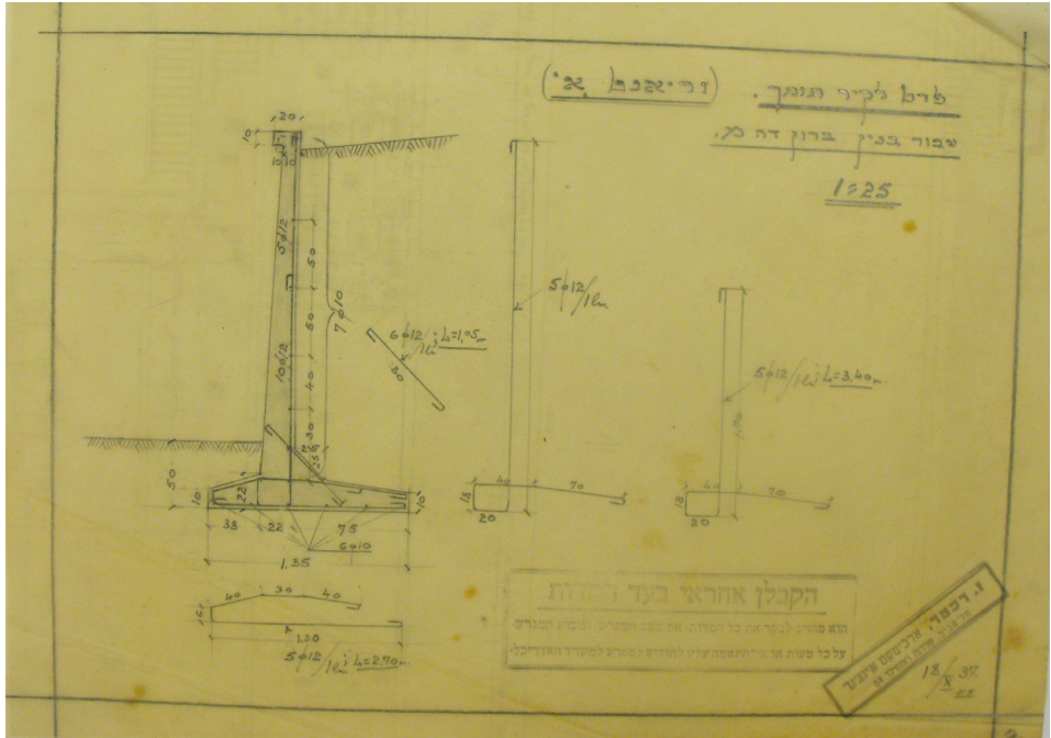
תוכנית רכטר לקירות התמך. מקור: ארכיון אמנון רכטר
