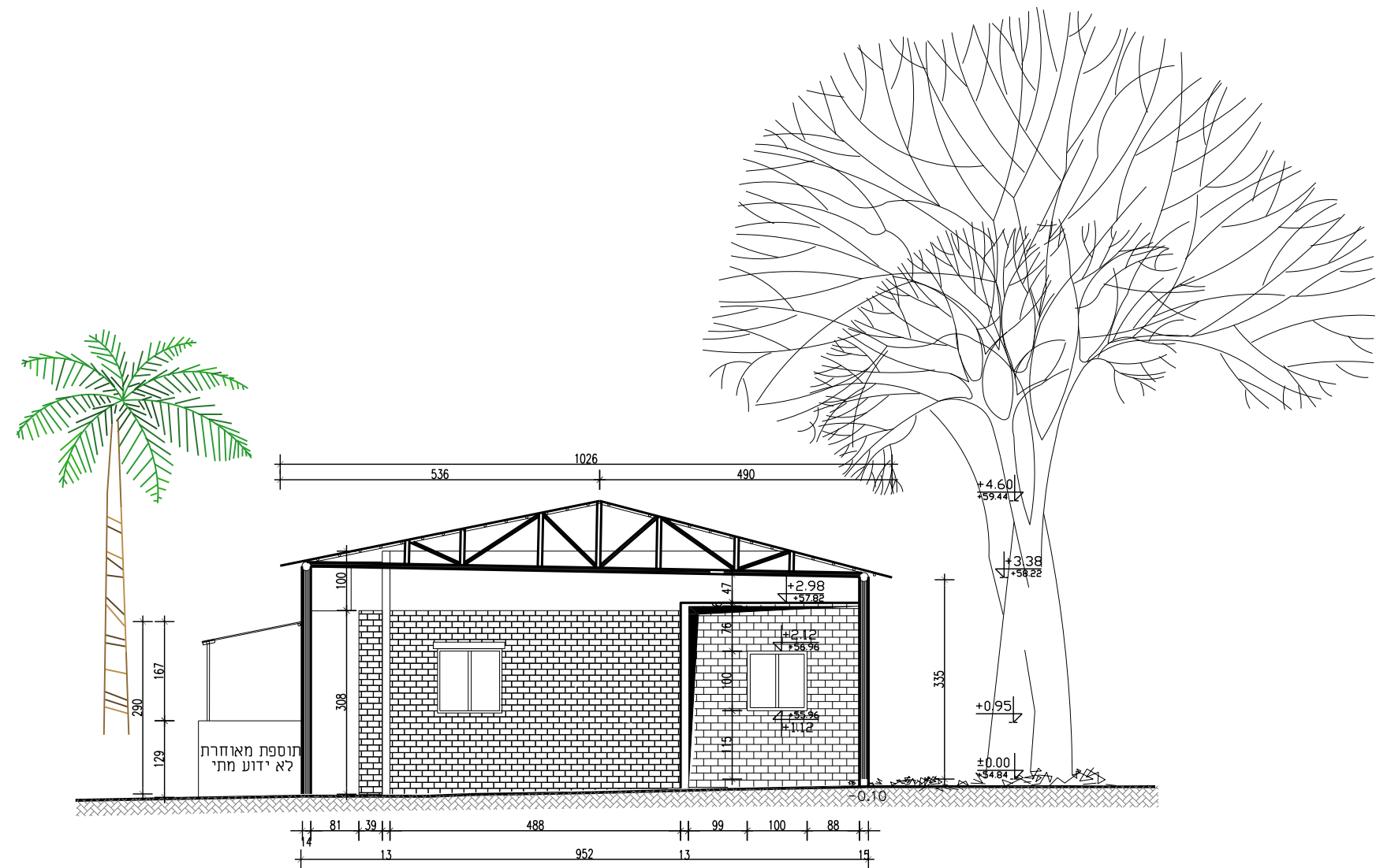
חזית צפון מערבית - מצב מקורי משוחזר - בית משפחת יפה קנה מידה 1:100
