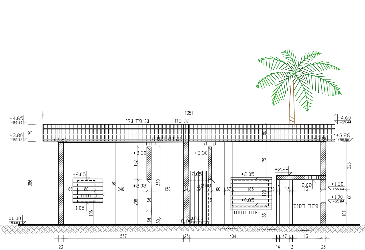
חתך א-א קנה מידה: 1-100
