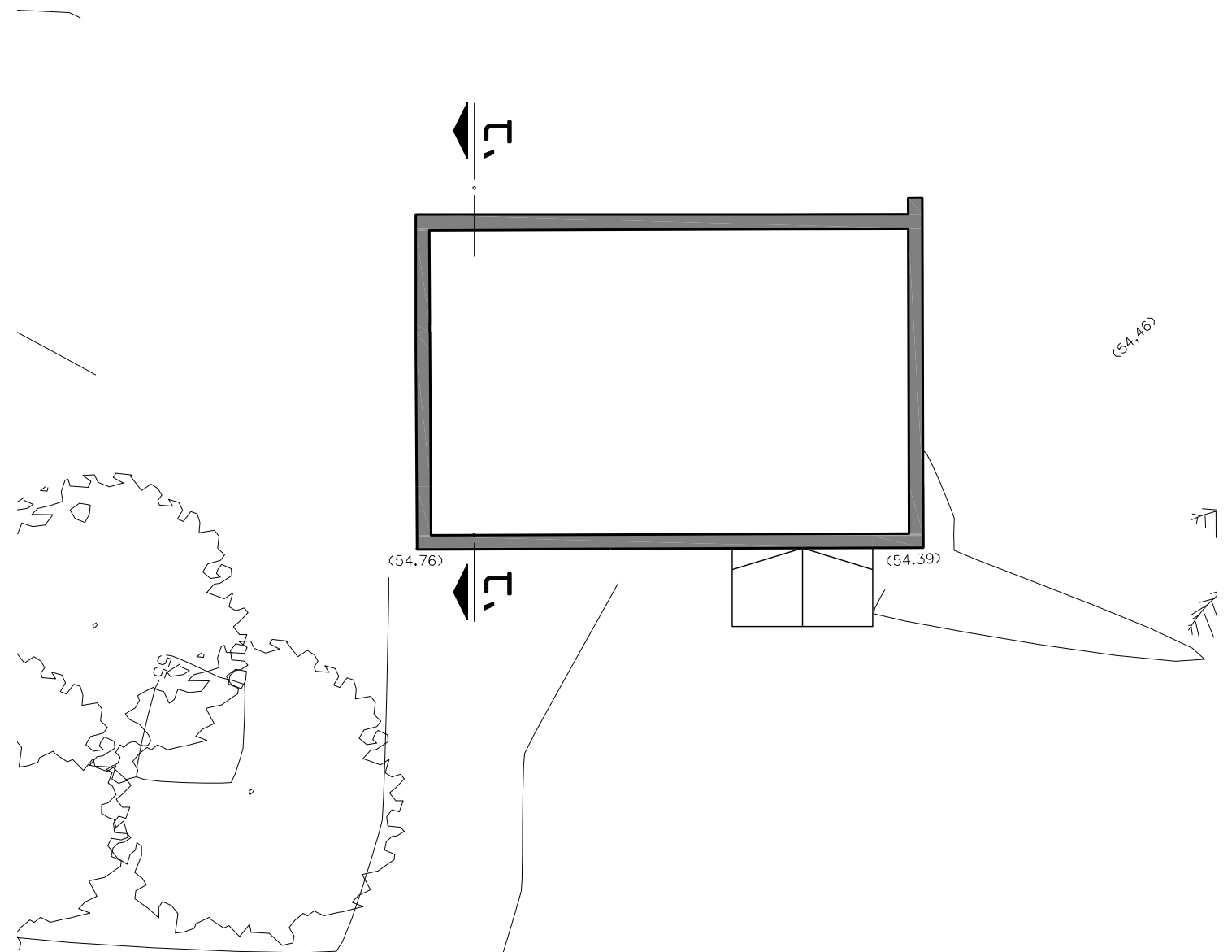
תוכנית קומת גג - מצב מקורי משוחזר - בית הנהג קנה מידה 1:100
